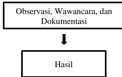
Gambar 1.1 Kerangka Teori
